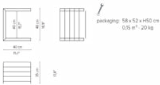
C-TABLE 01285
